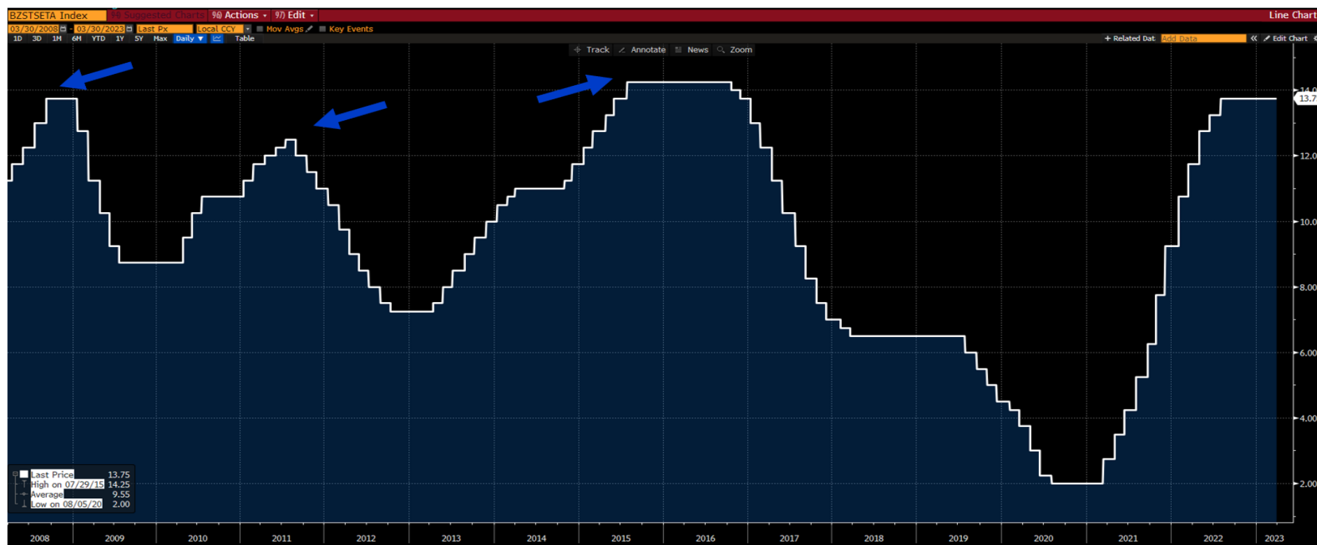
Taxa Selic Últimos 15 anos
