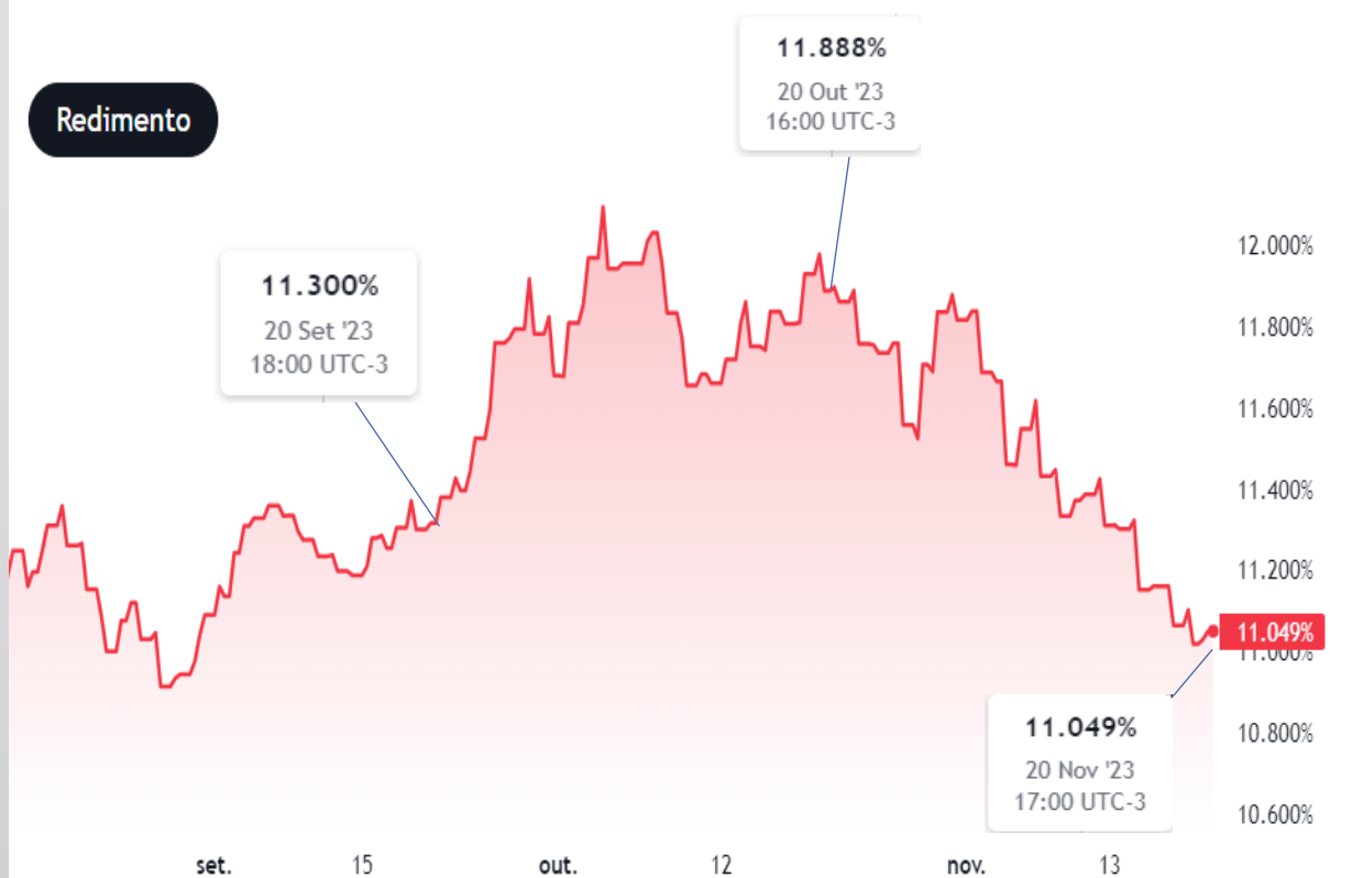
Gráfico de BR10Y >
